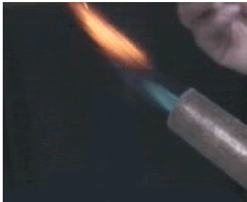
احتراق مسحوق الالومنيوم
